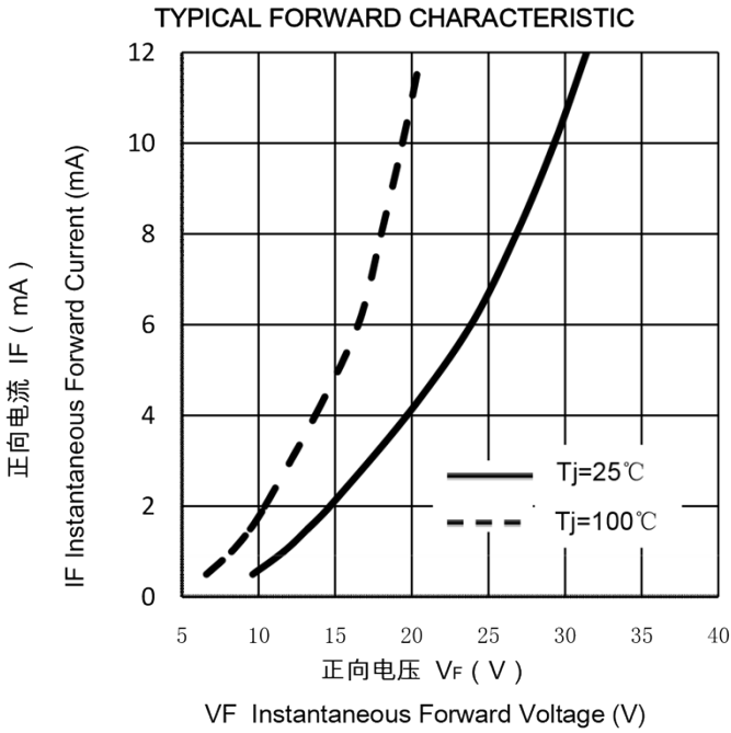
正向特性曲线 (典型值)
