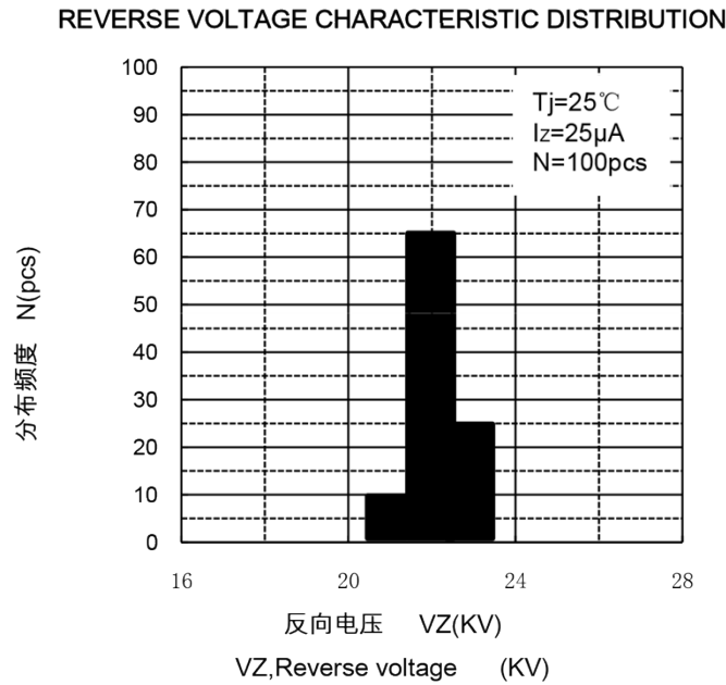
反向电压特性分布
