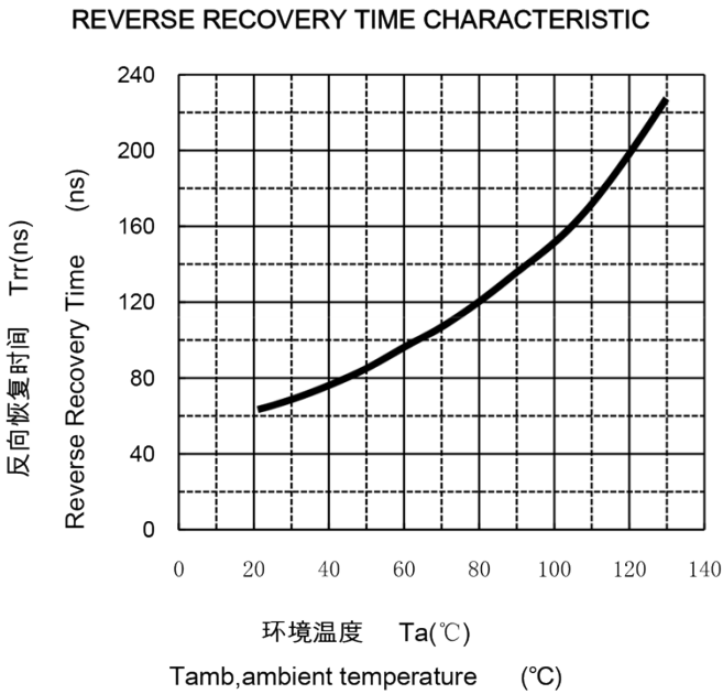
反向恢复时间特性
