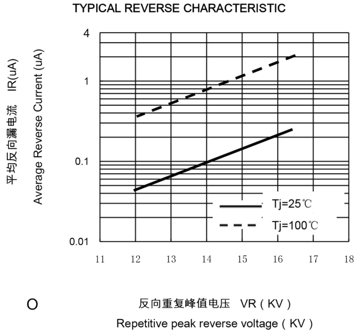
反向特性曲线
